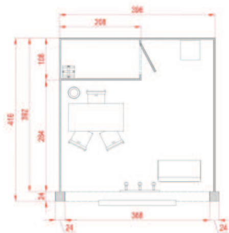
PIANTA - TIPO 16 mq
